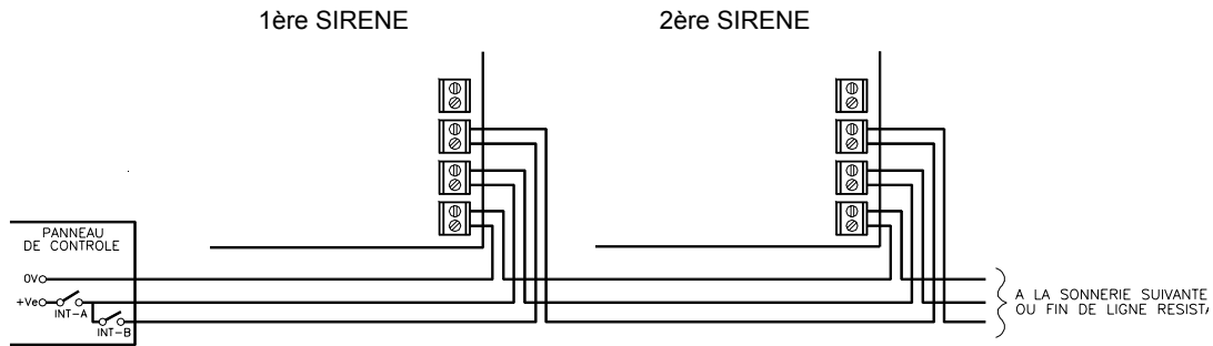
CABLAGE DES UNITES YL
