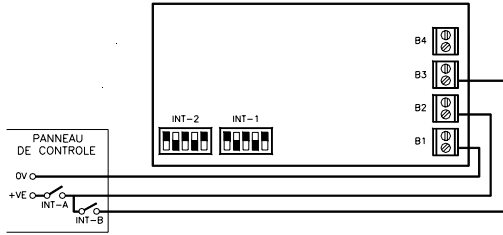
FIGURE 2: ENTREE DC - 2ème ETAPE PAR INVERSION DE L'ALIMENTATION
